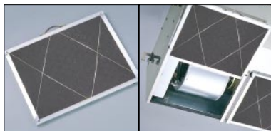
▲オイルミストフィルター ▲取手を引くだけのスライドアウト方式
