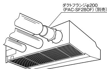
(外気取入用ロックアウト穴(φ200) P80形…2ヵ所、P140形…3ヵ所)
